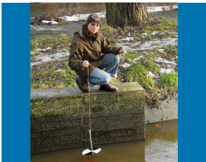
Měření průhlednosti vody Secchiho deskou
